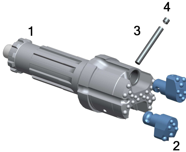
PCON-E 180 组件表
