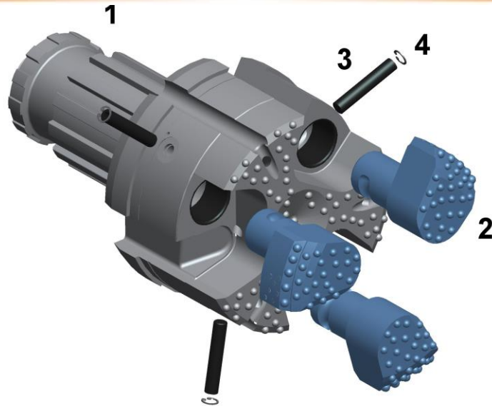
PCON-E 365 组件表
