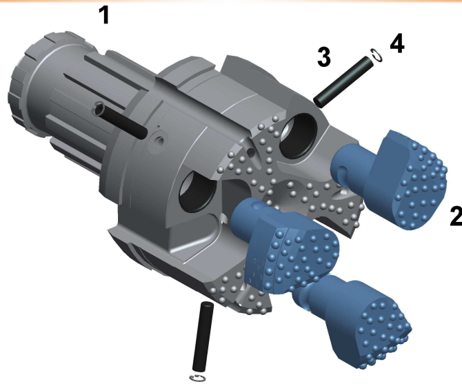
PCON-E 510 组件表
